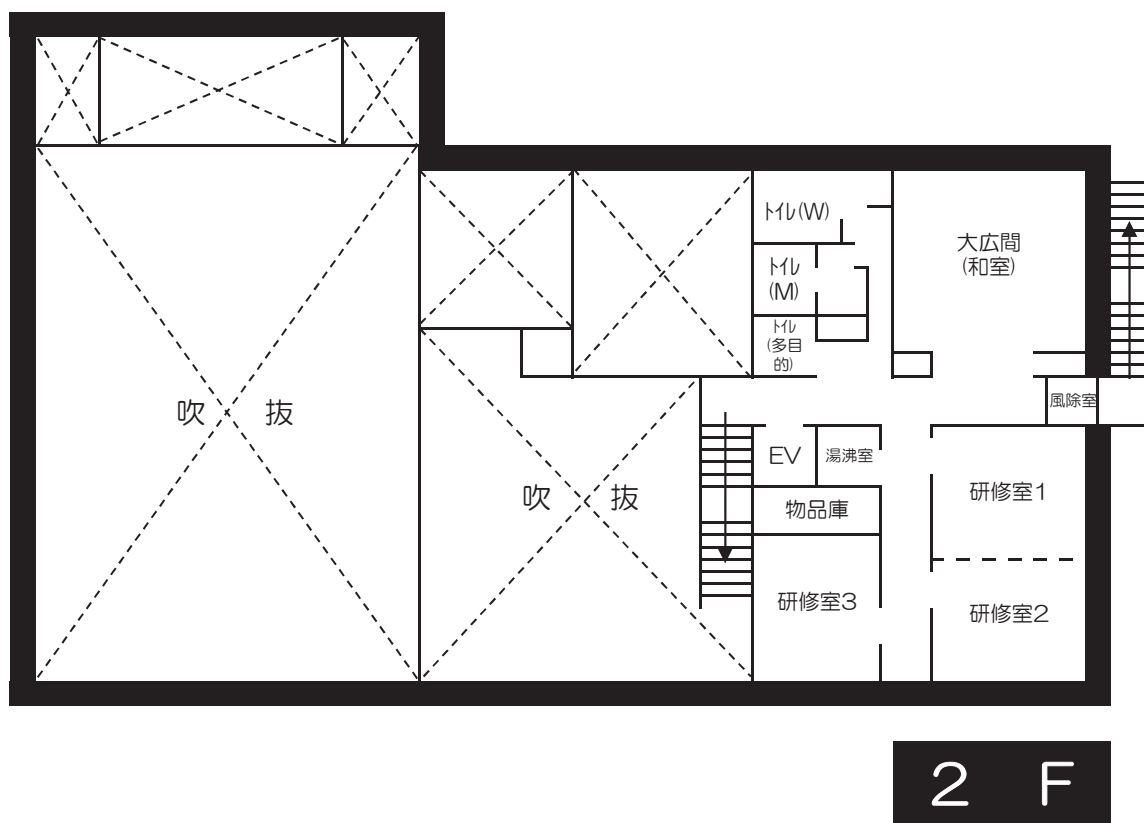
木野コミュニティセンター 平面図
